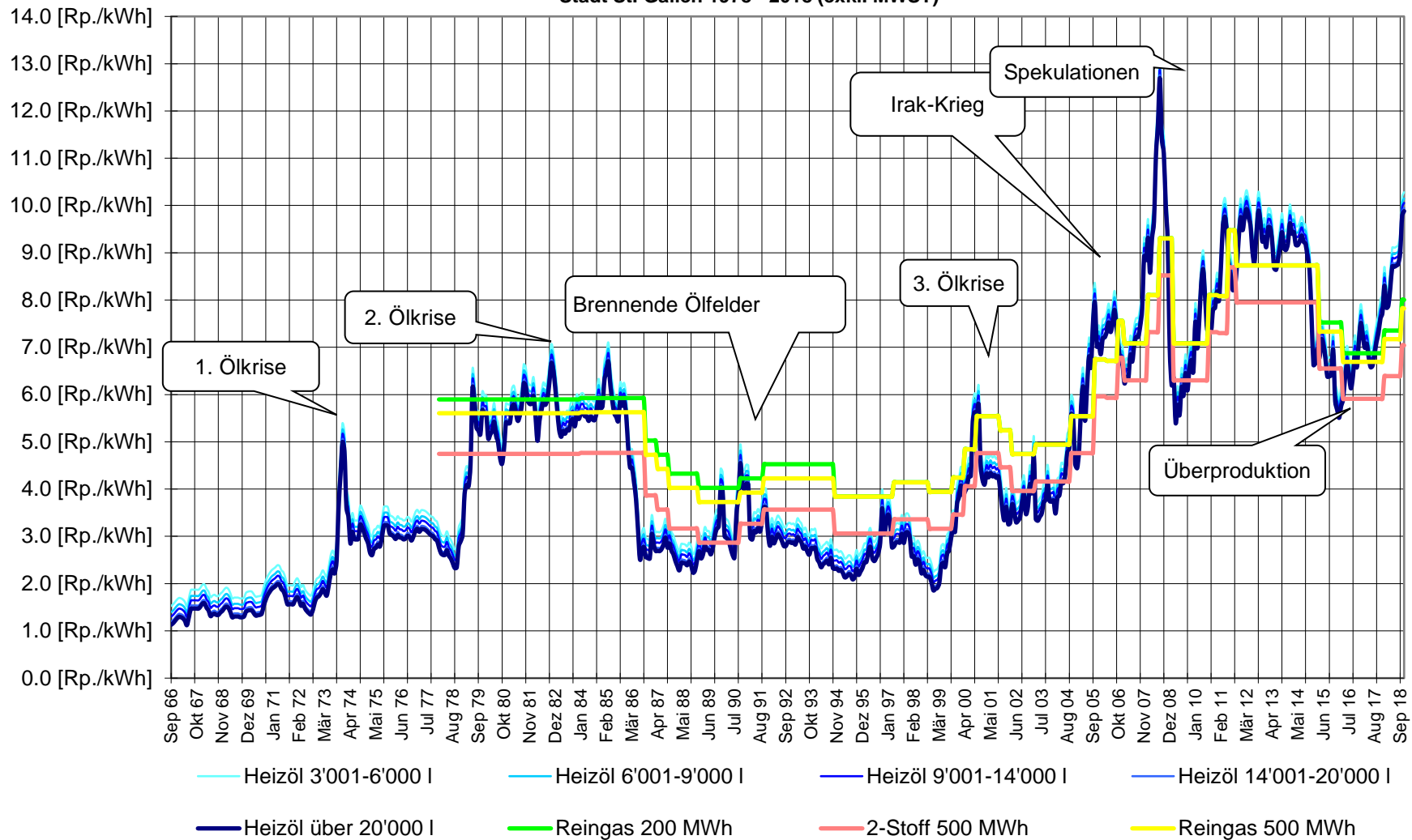
Erdgaspreise / Heizölpreise EL für 3'000 bis über 20'000 Liter, Reingas EG1 / 2-Stoff EG2 Stadt St. Gallen 1978 - 2018 (exkl. MWST)
