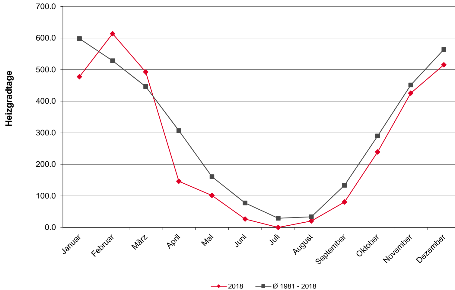
Heizgradtage Schellenacker St.Gallen (20/16°C)
