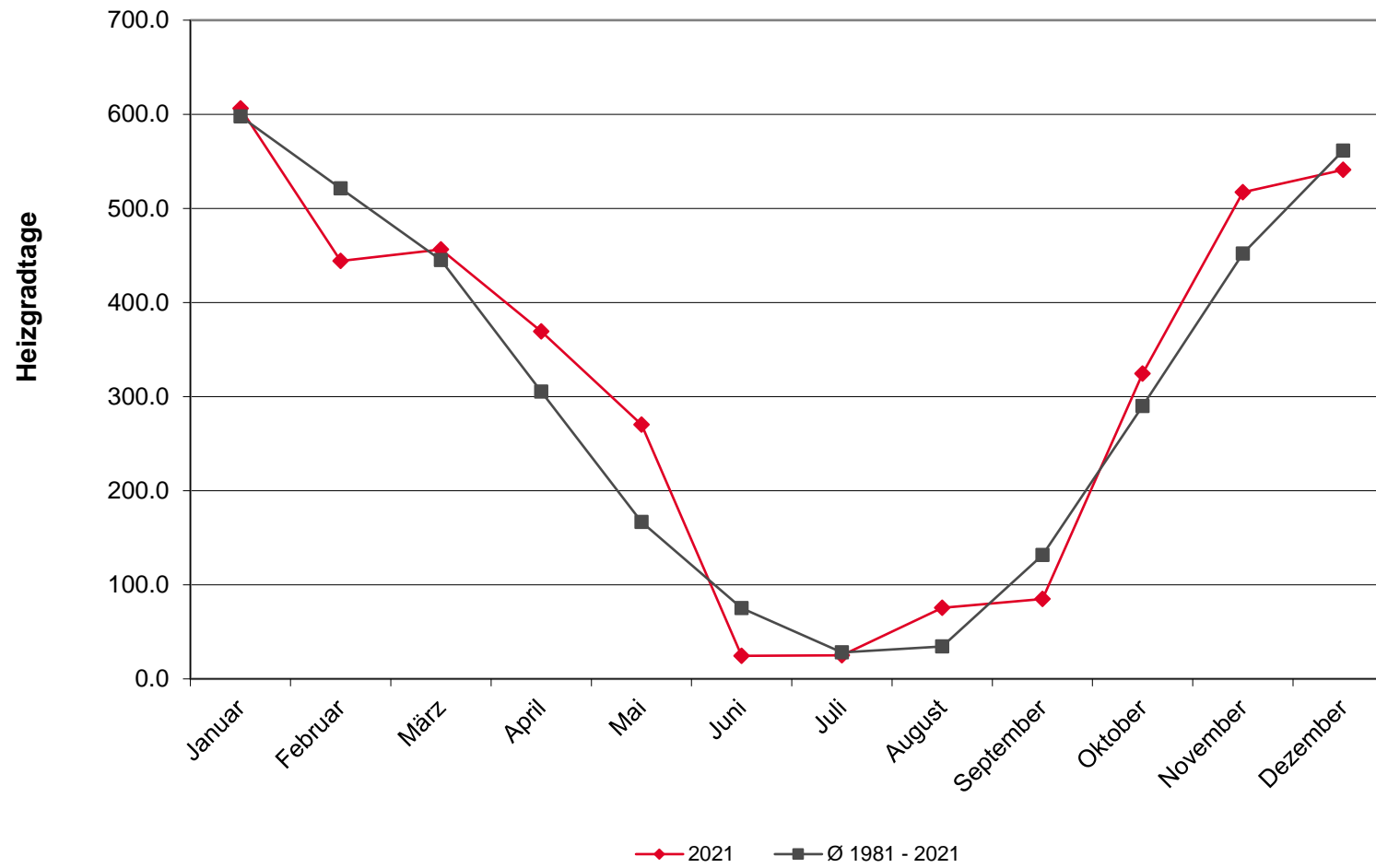
Heizgradtage Schellenacker St.Gallen (20/16°C)
